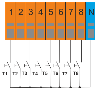
Anschluss Taster
