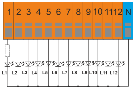
Anschluss LEDs
